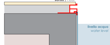
Guida sotto bordo Under edge guide
