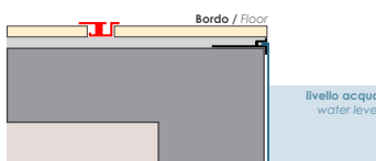
Guida a scomparsa Hidden guide
