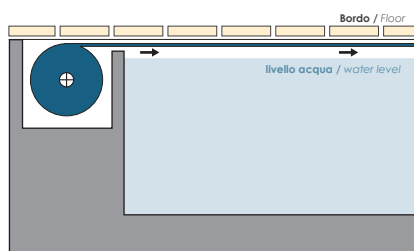
CONFIGURAZIONE - C Vano motore interrato con guide sotto bordo Underground compartment and under edge guides
