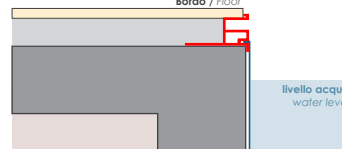
Guida sotto bordo Under edge guide
