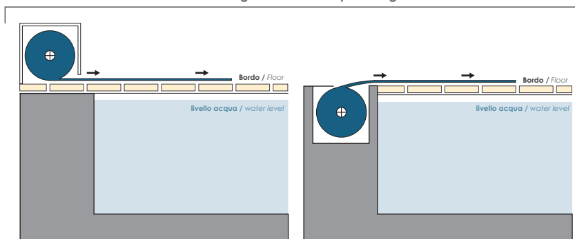
CONFIGURAZIONE - A Vano motore fuori terra con guide sopra bordo External compartment and external guides
