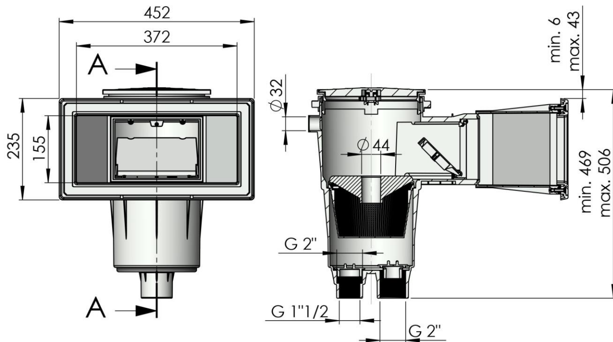
SECCIÓN A-A
