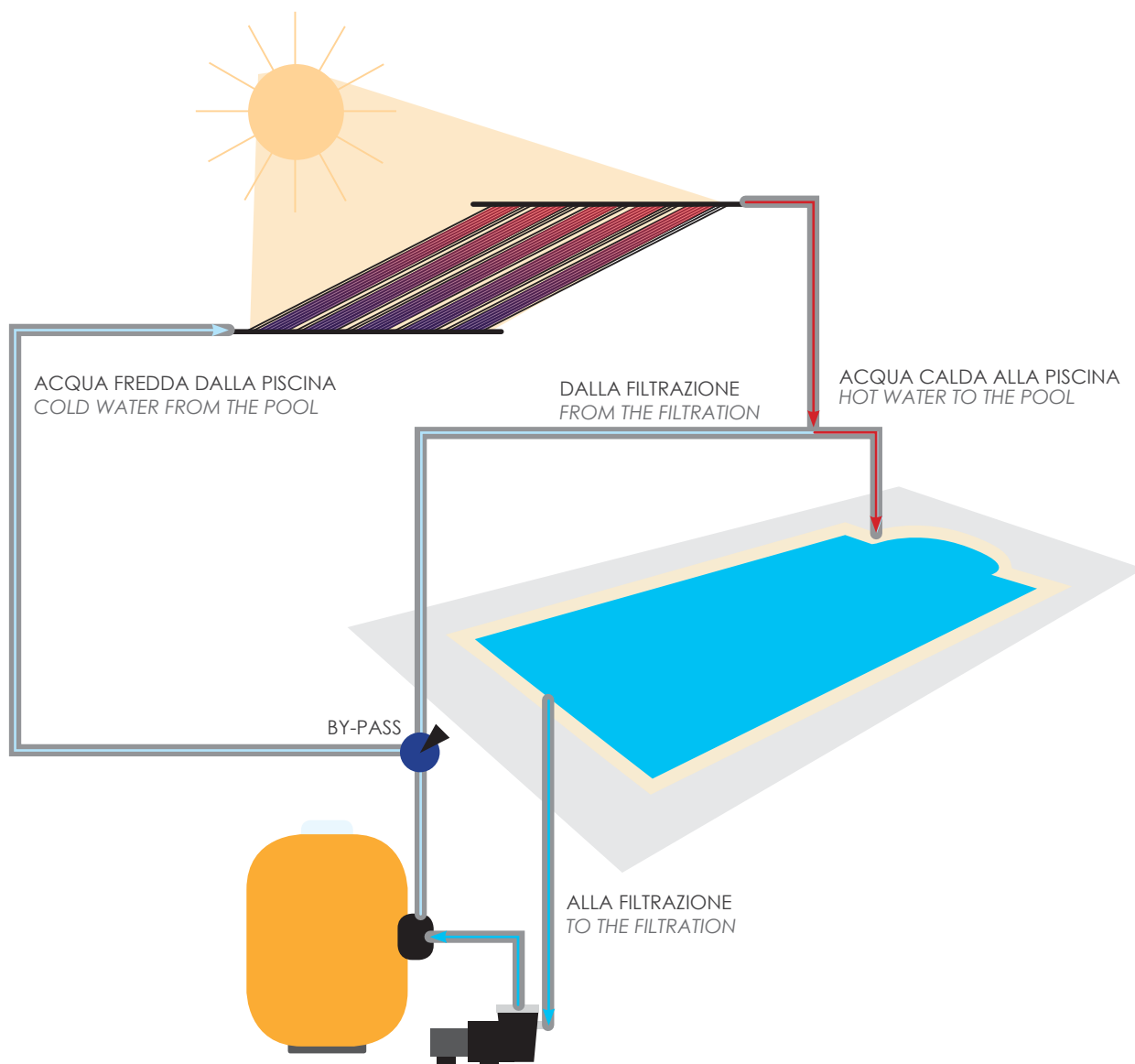
Fig 7: Collegamento del pannello solare al sistema Fig 7: Joint panel-system
